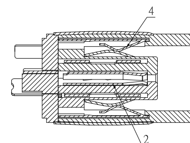
SECTION B-B 旋轉45°
