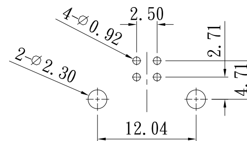
PCB LAYOUT(SCALE:2X)
