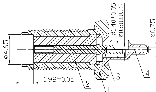
A-A剖視圖 CD000952002-3 小SMA母頭(母PIN)FOR \phi 0.8 -組件
