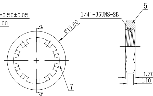
A-A剖視圖 銅墊圖 CD013922002-4
