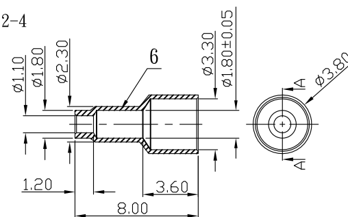
A-A剖視圖 CD000952002-2 小SMA母頭(母PIN)FOR \phi 0.8 -后套
