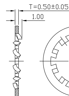
A-A剖視圖 銅墊圖 CD013922002-4
