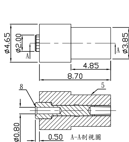
小SMA公頭(母PIN)-組件2
