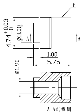
小SMA公頭(母PIN)-本體B
