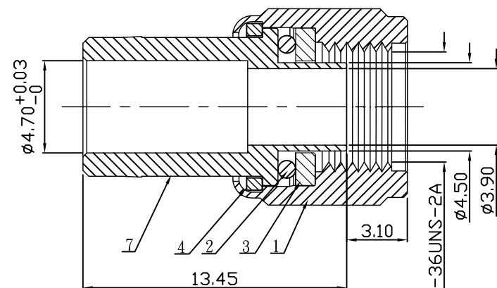
A-A剖視圖(裝配)
