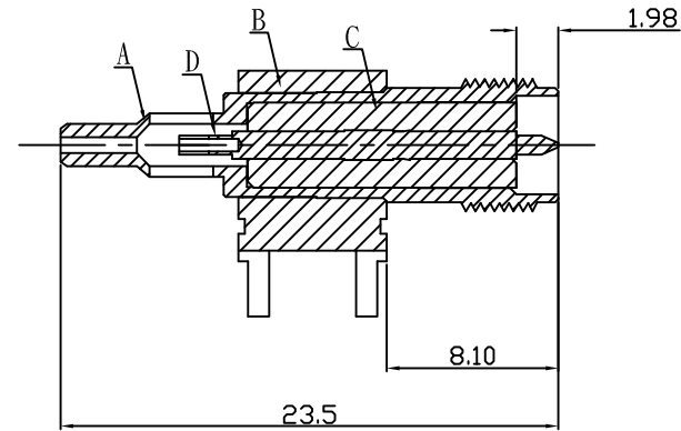
A-A剖視圖
