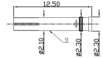
SCALL:2:1 CD013922005-8
