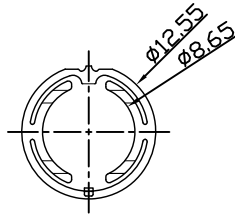
SCALL:2:1 CD013922005-6
