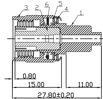
CD013922005-9(組件)
