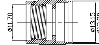
A-A部剖視圖 CD013922005-2
