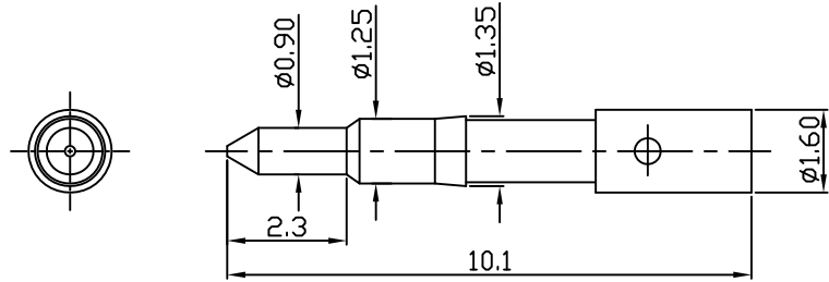
SMA母頭 (公PIN)-中心針 CD028922005-1
