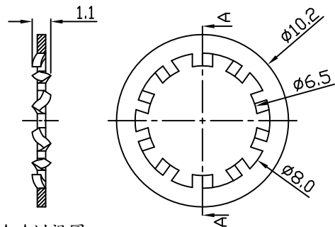
A-A剖視圖
