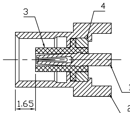
A-A' 剖面
